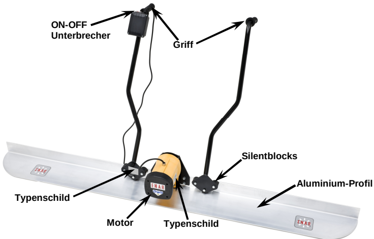
VIBRIERPATSCH MIT ELEKTRISCHEM ODER BENZINMOTOR "QX"
